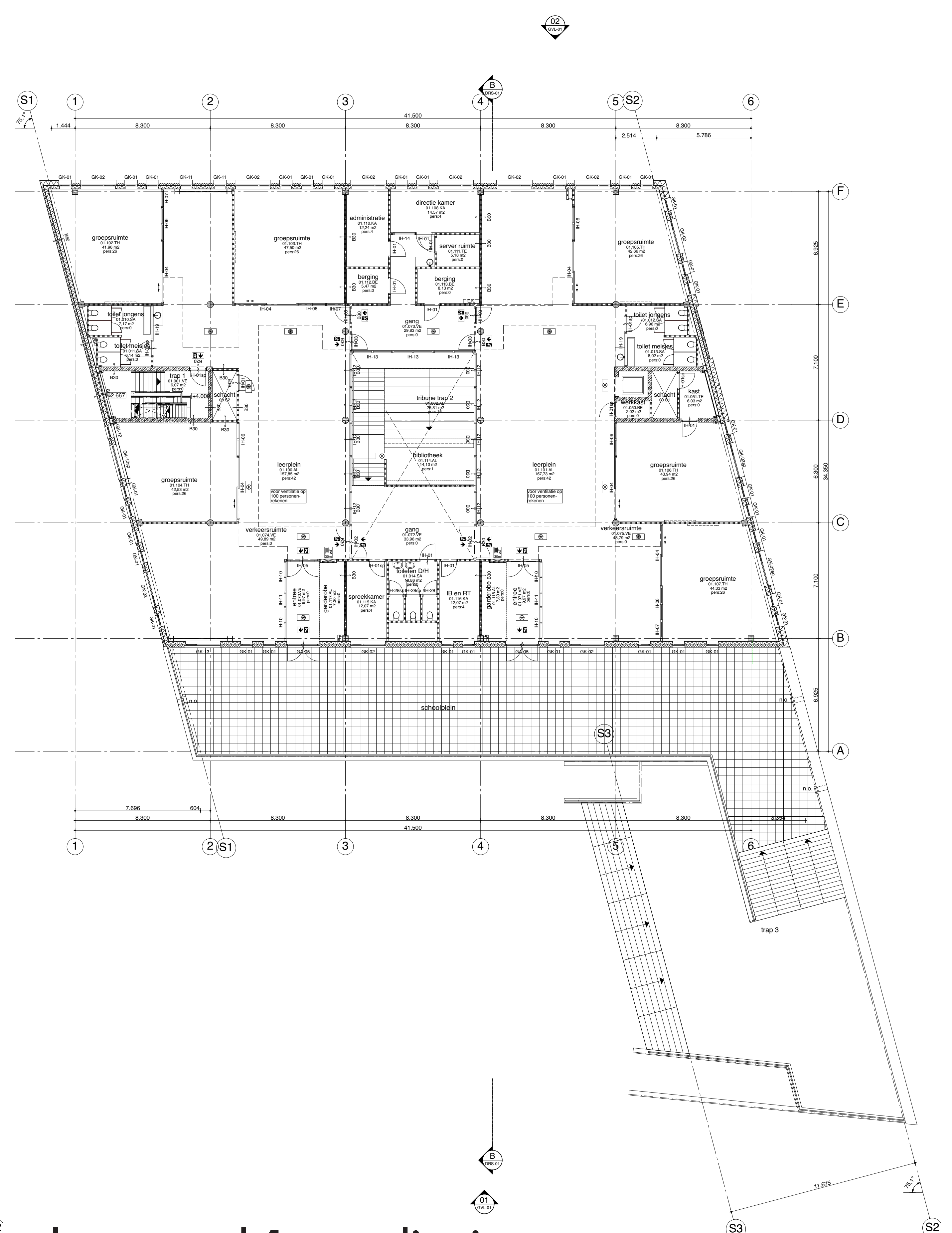
plattegrond 1e verdieping
