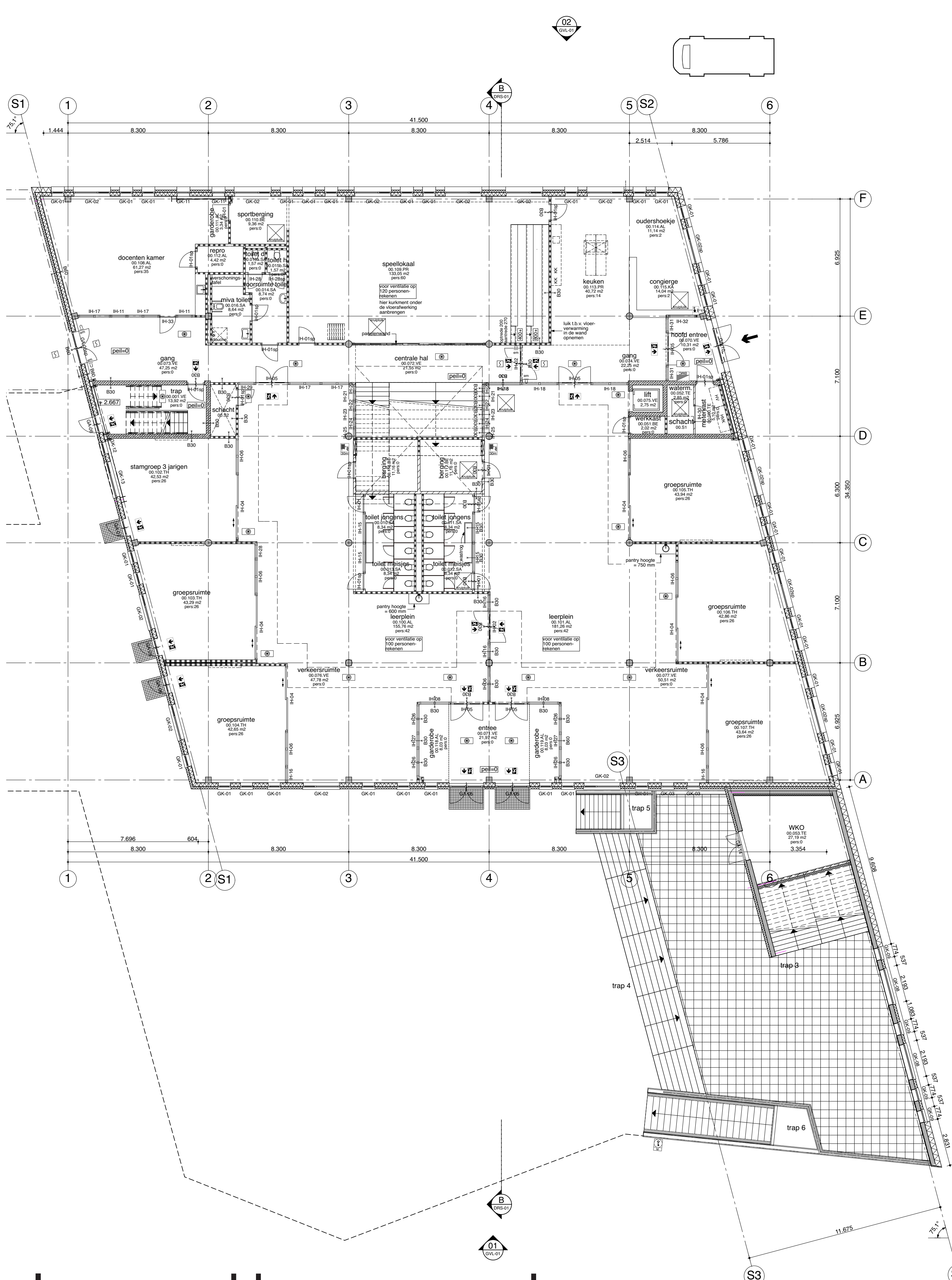
plattegrond begane grond
